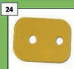
Katalogové číslo J52720000 Název výrobku Drák luční brány Použití Jaskin Ceníková cena 45,- Kč bez DPH / ks
