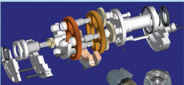
Excentrické převodovky typu EC Box
